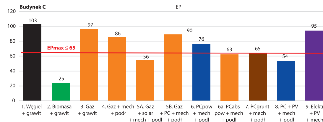
Rys. 4. Wskaźniki EP [kWh/m 2 a], które osiąga budynek C (wielorodzinny o pow. 526 m 2 ) dla każdego wariantu instalacji
